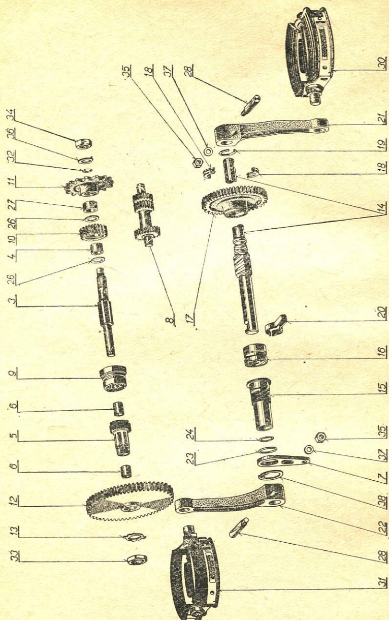
Transmission - Getriebe - Mécanisme de transmission - Transmisiones
