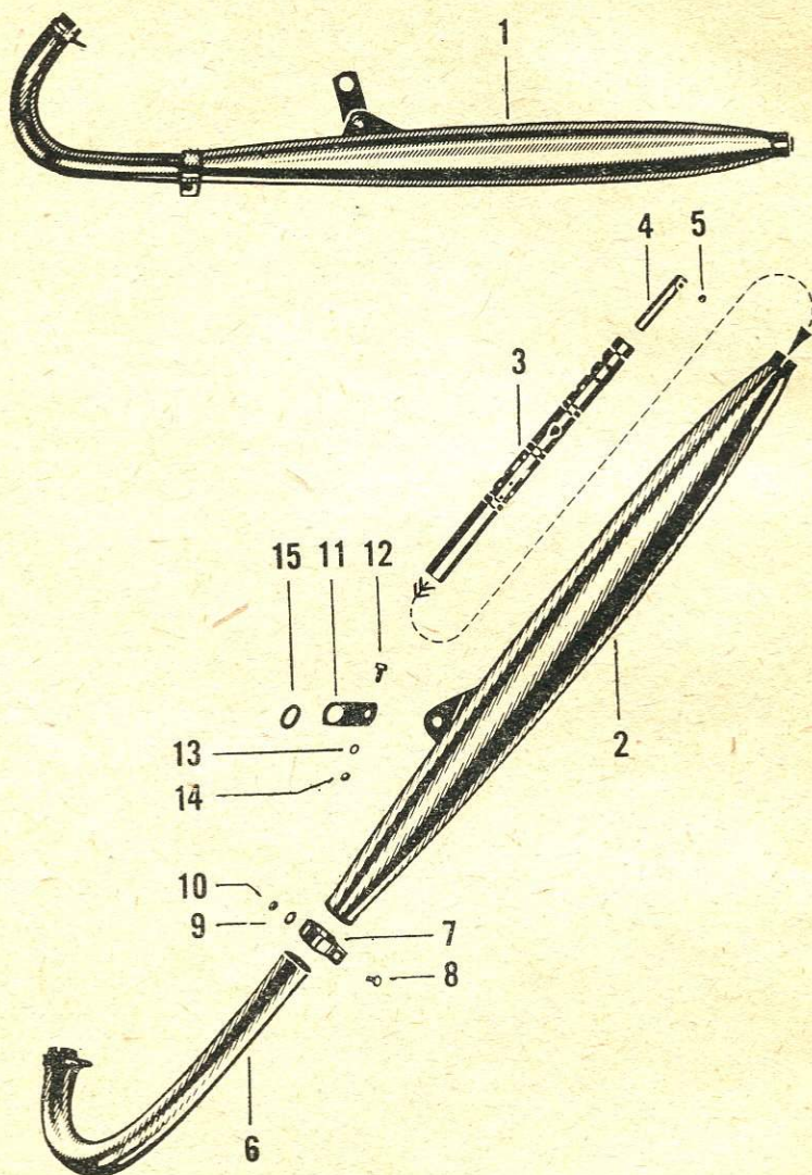
Exhaust Pipe and Silencer - Auspuffrohrleitung und Auspufftopf Tube d'échappement avec silencieux - Tubería de escape y silenciador de escape
