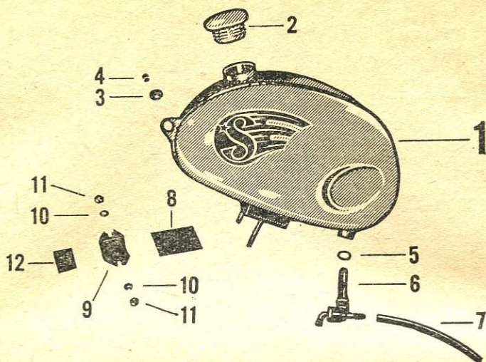
Fuel Tank - Kraftstoffbehälter - Réservoir de carburant - Tanque de combustible
