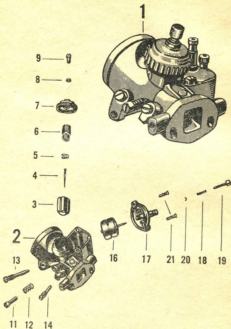
Carburettor Jikov - Vergaser Jikov - Carburateur Jikov - Carburador Jikov
