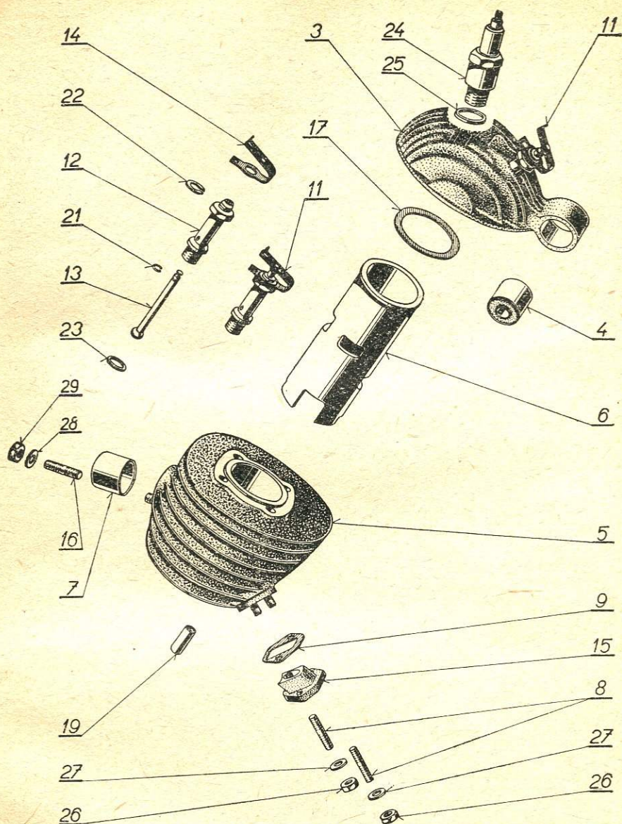
Cylinder Barrel with Cylinder Head - Zylinder mit Zylinderkopf - Cylindre avec culasse - Cilindro con culata
