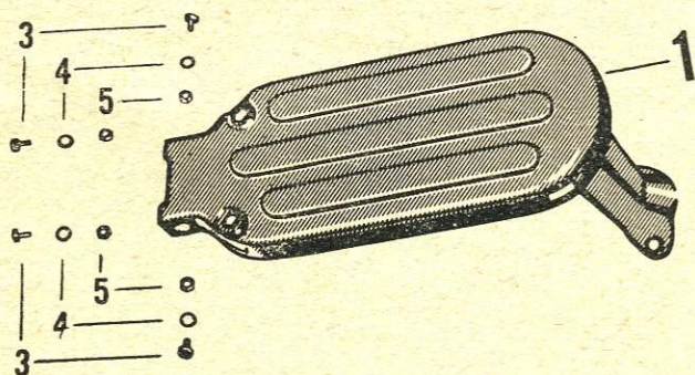
Luggage Carrier - Gepäckträger - Porte-bagage - Portaequipajes
