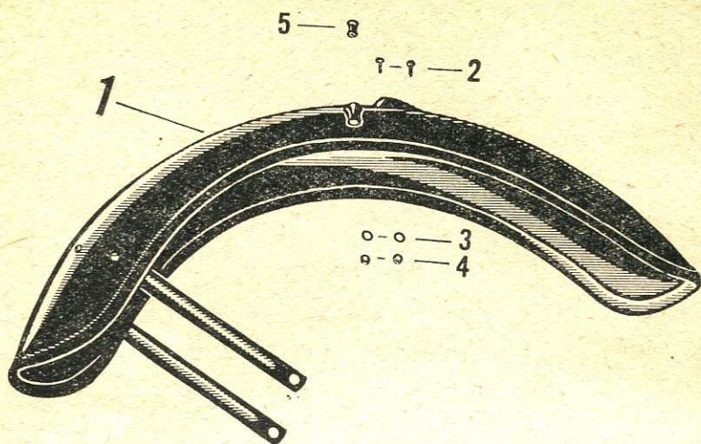
Front Wheel Mudguard - Vorderer Kotflügel - Garde-Boue AV - Guardabarros delantero
