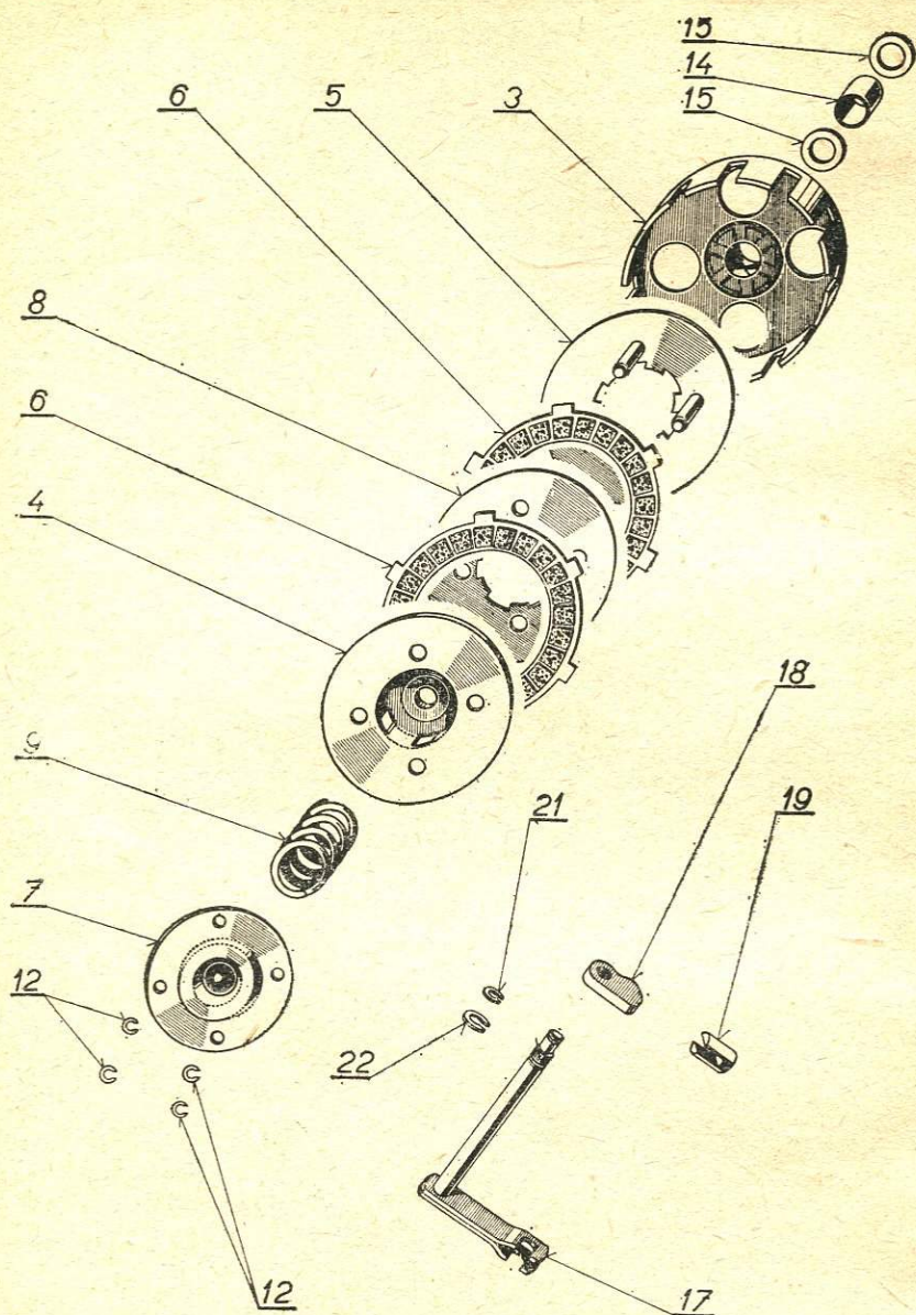
Clutch Complete - Komplette Kupplung - Embrayage - Embrague completo
