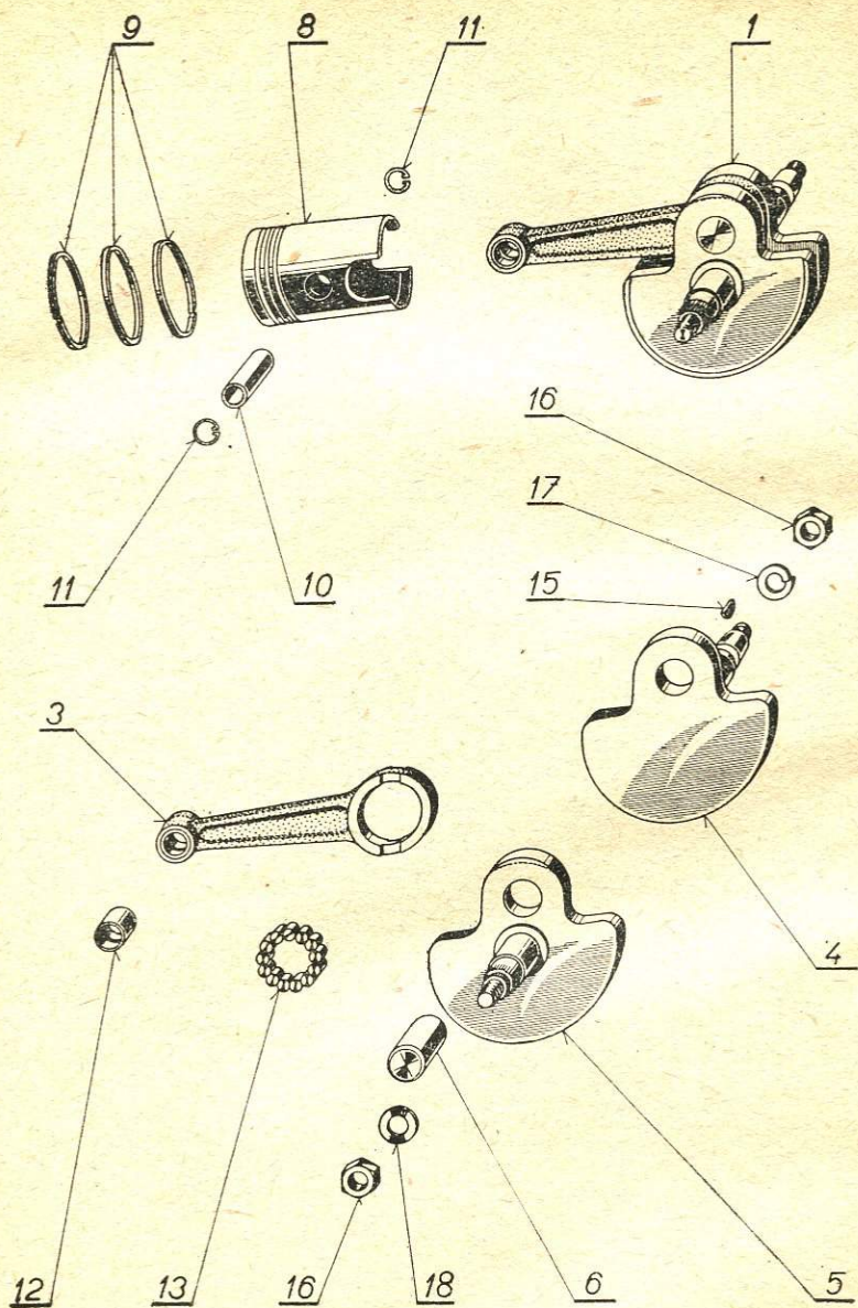
Crankshaft Mechanism - Kurbeltriebwerk - Attelage moteur - Mecanismo de biela
