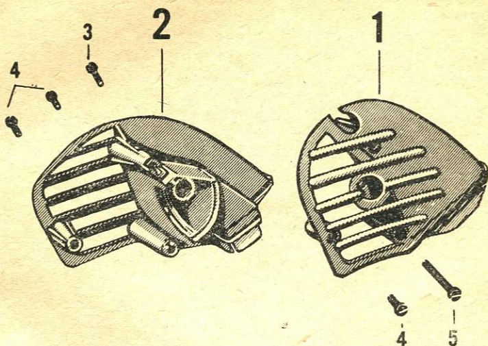
Intake Silencer - Ansaugdampfer - Silencieux d'admission - Silenciador de aspiración
