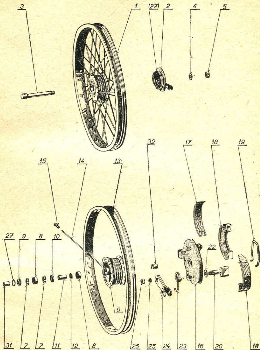
Front Wheel - Vorderrad - Roue AV - Rueda delantera
